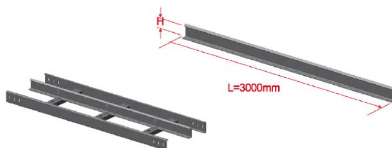
BL*-D N*-D Divider
