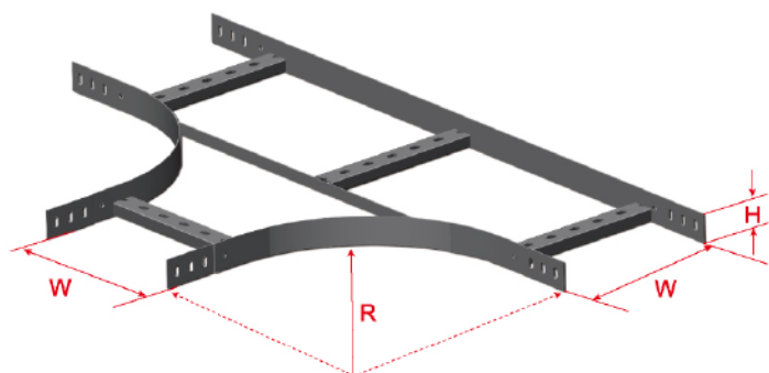
BL2-T Tee
