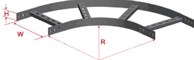
BL2-E Elbow 90°
